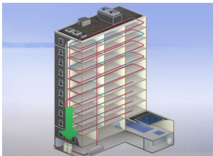
중앙집중식 급탕 설비의 예
